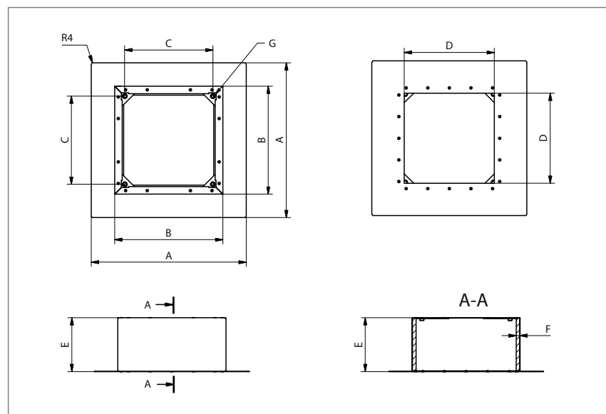
wymiary oraz przykład montażu podstawy DSK
