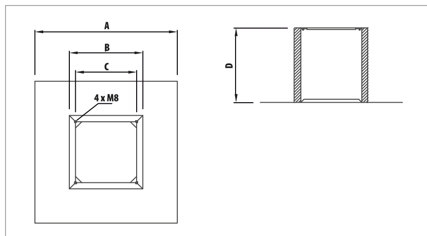
wymiary oraz przykład montażu podstawy DSF AL i akcesoriów
