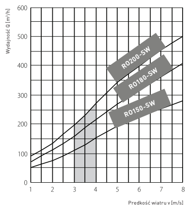
Wykres wydajności samonastawnych nasad kominowych ROTOWENT DRAGON w zależności od prędkości wiejącego wiatru bez uwzględnienia wysokości kominu.
